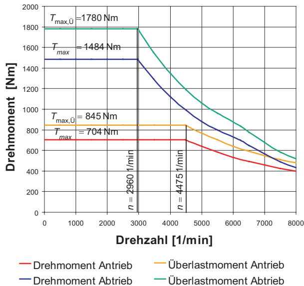
Abb. 1: Motorkennfelder der Asynchronmaschinen
