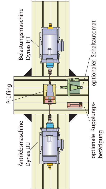
Abb. 2: Prinzipieller Prüfstands Aufbau mit Antriebsstrang, Prüfling und Abtriebsstrang
