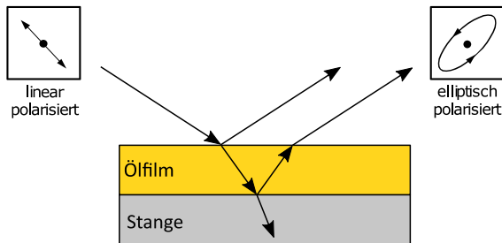
Prinzipskizze
