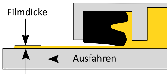
Schmierfilmdicke
